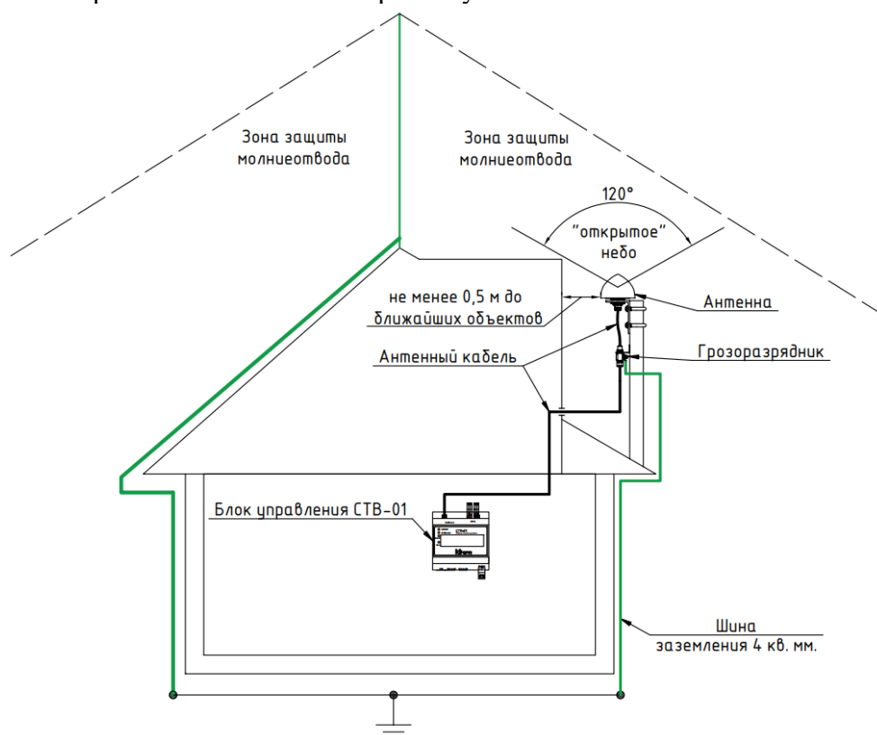
Рисунок 3.1.1 Схема размещения антенны и грозоразрядника.
