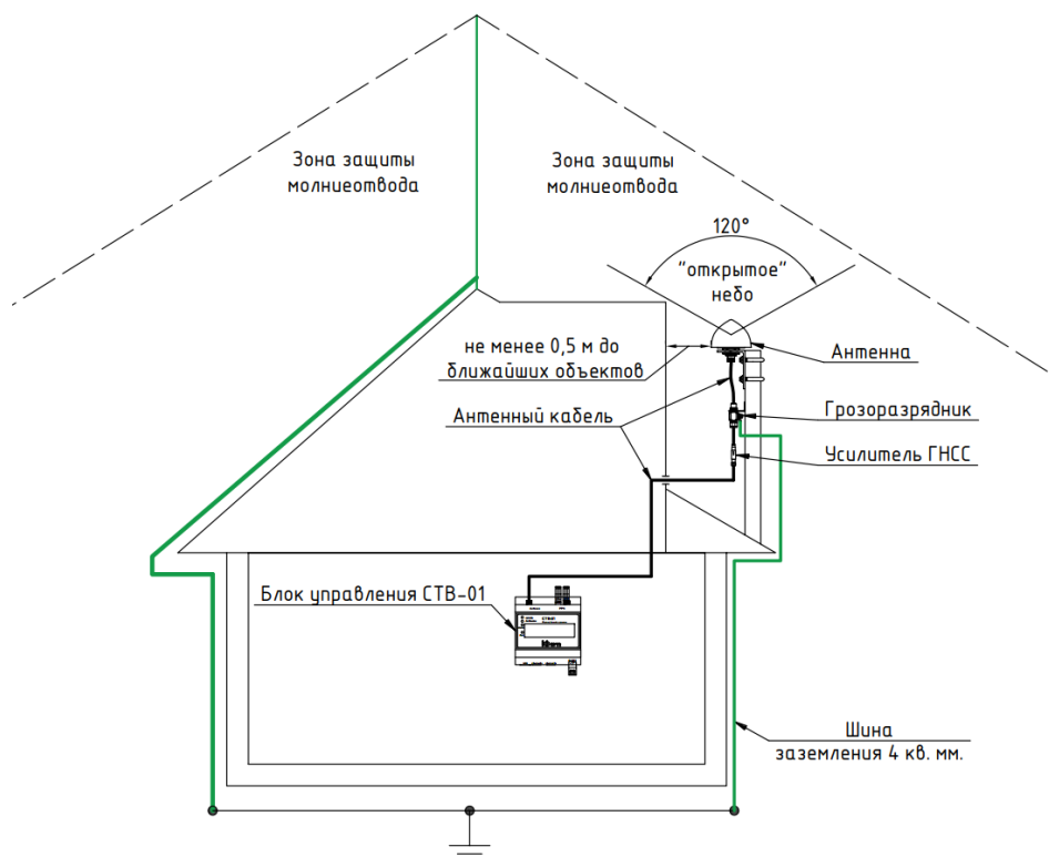
Рисунок 3.1.2 Схема размещения антенны, грозоразрядника и усилителя ГНСС (опционально).
