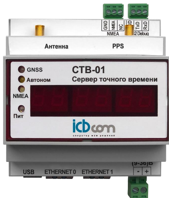
Рисунок 2.2.2. Передняя панель блока управления СТВ-01 (DIN) с ревизией корпуса P2.
