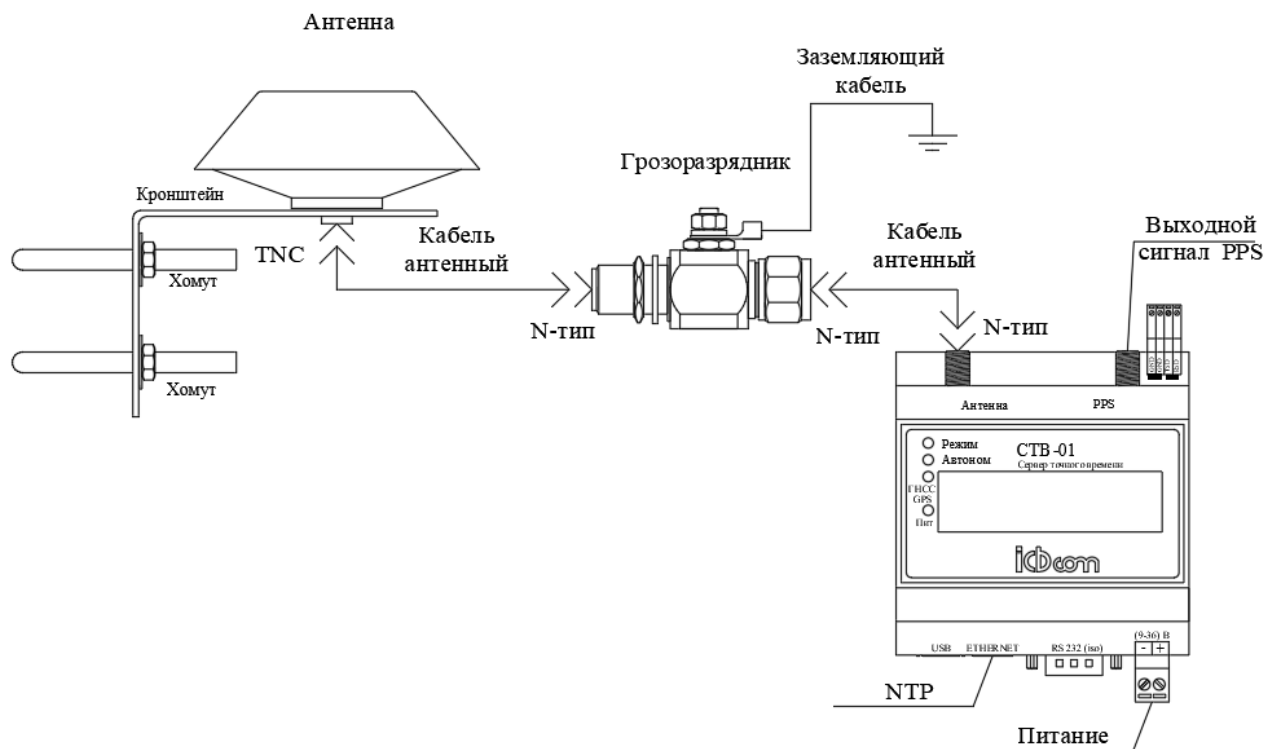
Рисунок 3.2.1.1 Схема соединения узлов СТВ-01 (DIN) с ревизией корпуса P1 с грозозащитником.
