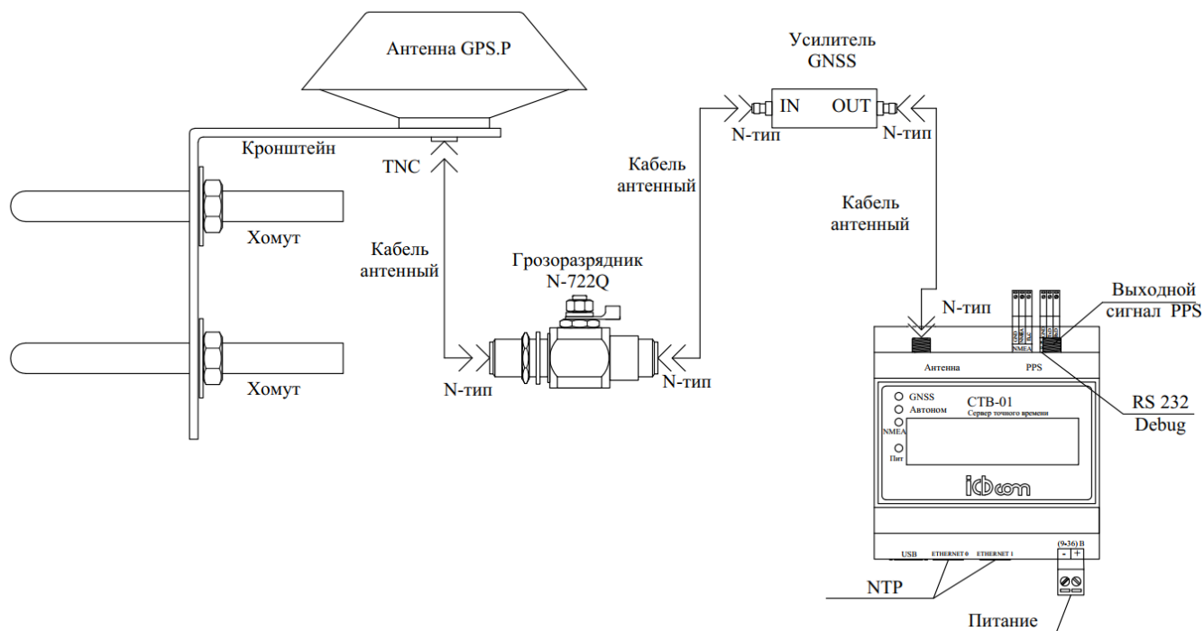
Рисунок 3.2.2.2 Схема соединения узлов СТВ-01 (DIN) с ревизией корпуса P2 с грозоразрядником и усилителем ГНСС (опционально).
