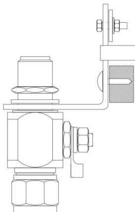
Рисунок 3.3 Крепление грозозрядника.
