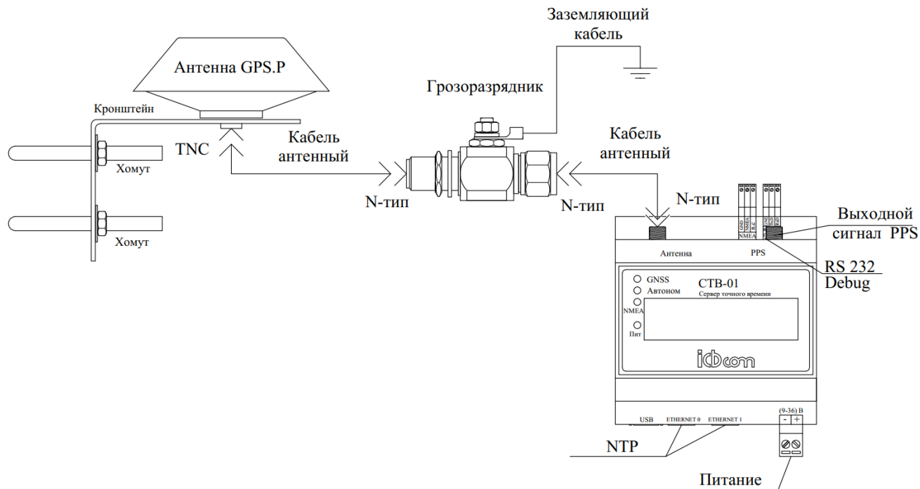
Рисунок 3.2.1.2 Схема соединения узлов СТВ-01 (DIN) с ревизией корпуса P2 с грозозащитником.
