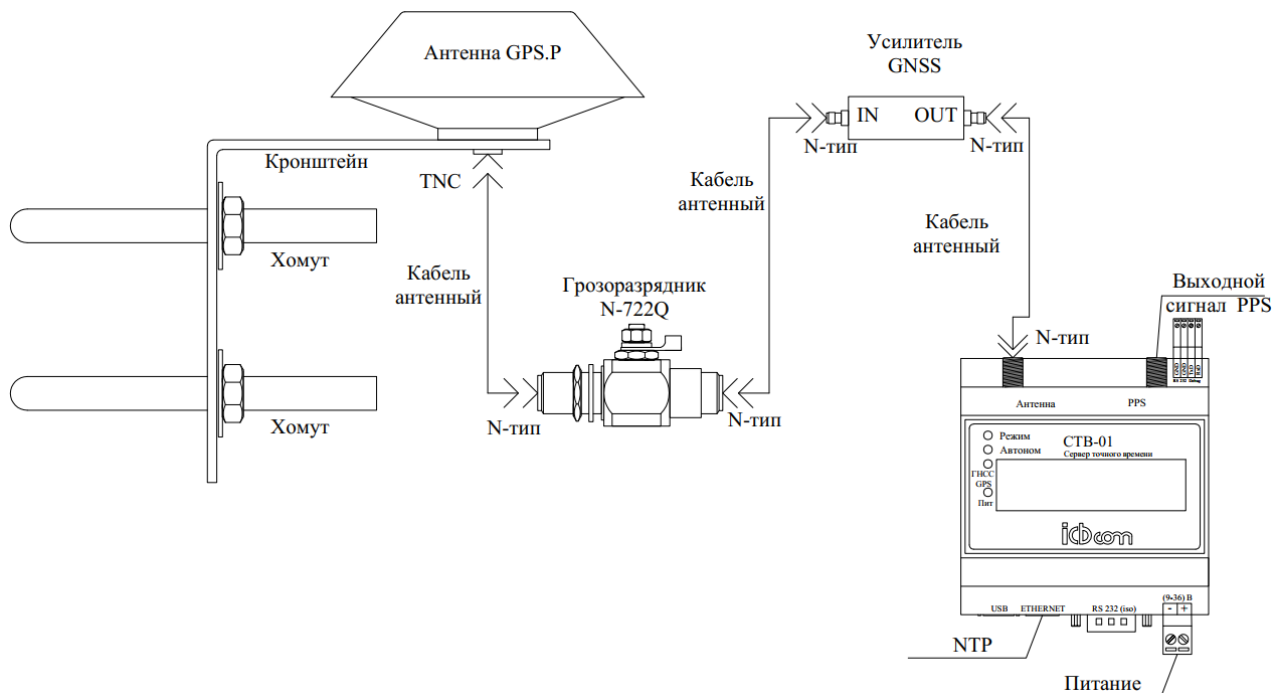
Рисунок 3.2.2.1 Схема соединения узлов СТВ-01 (DIN) ревизией корпуса P1 с грозоразрядником и усилителем ГНСС (опционально).
