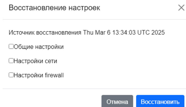
Рисунок 47 – Окно Recovery.
