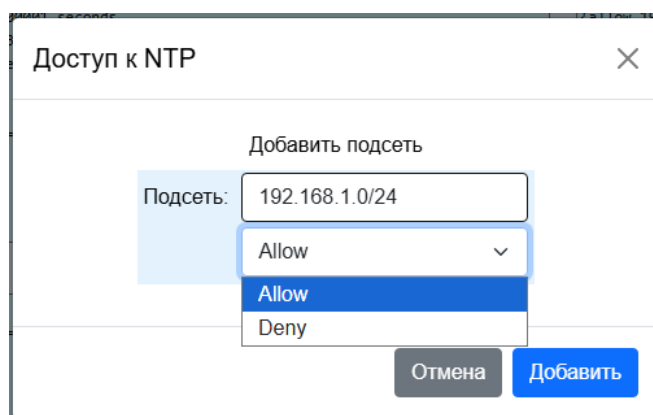
Рисунок 17 – Добавление подсети.
