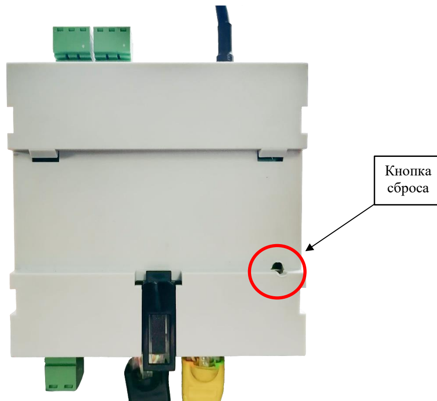
Рисунок 2.3. Задняя панель блока управления СТВ-01 (DIN) с ревизией корпуса Р2.
