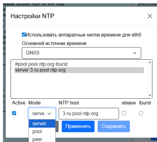
Рисунок 13 – Настройки дополнительных источников синхронизации NTP.
