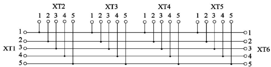
Рисунок 2 – Схема электрическая принципиальная
