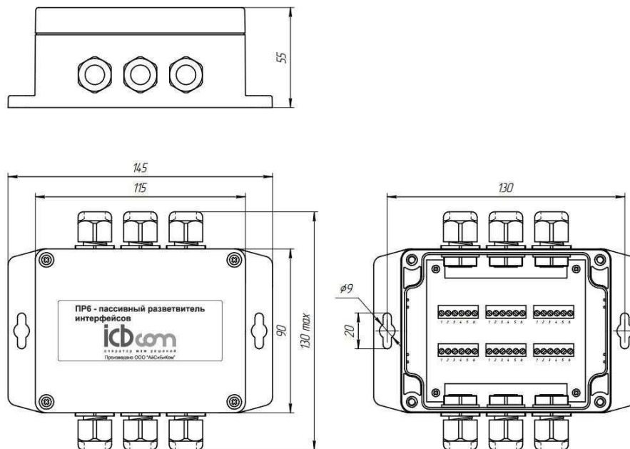
Рисунок 3 – Габаритные размеры
