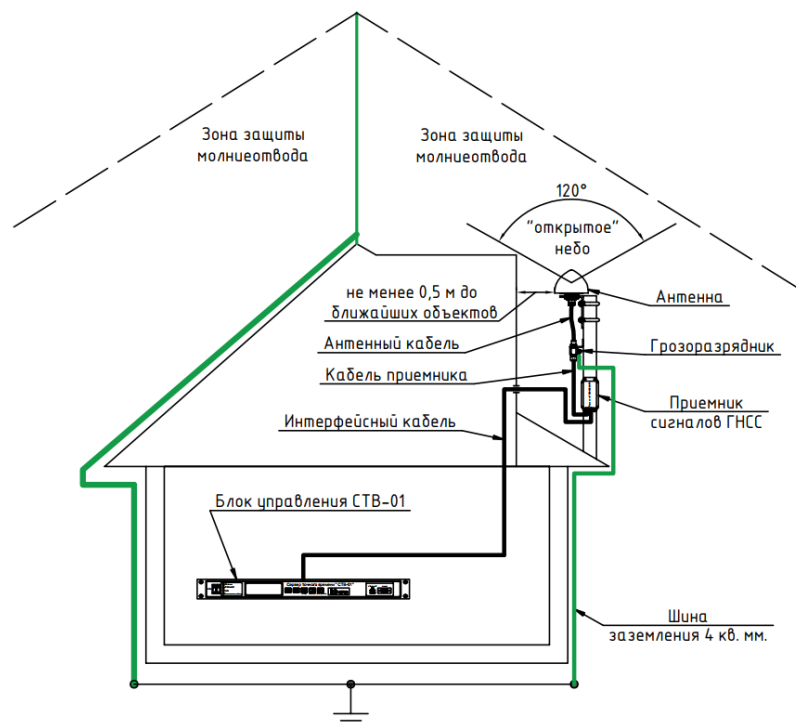
Рисунок 3.1 Схема размещения антенны на трубе. Схемы соединения узлов представлены на рисунках 3.2.
