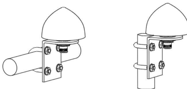
Рисунок 3.4 – Крепление антенны.
