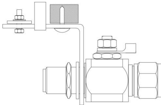
Рисунок 3.3 – Крепление грозоразрядника.
